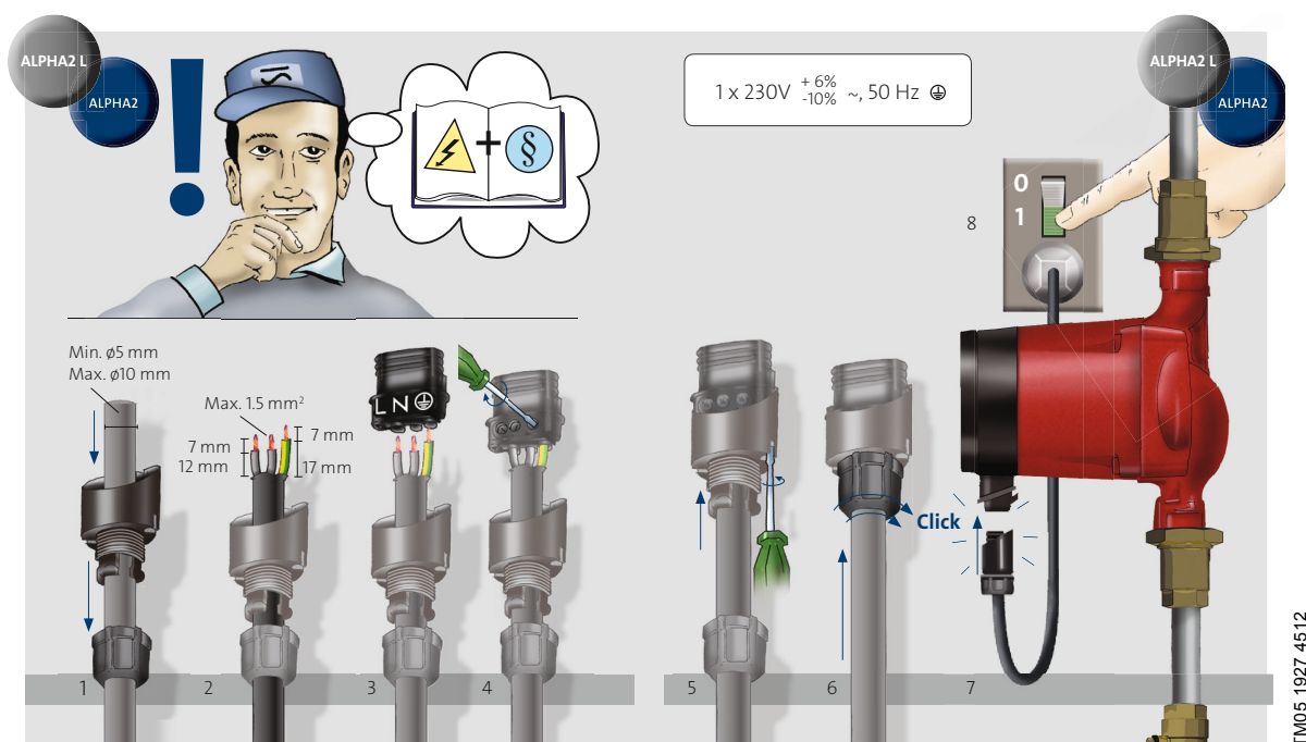
Obr. 6 Elektrické připojení
